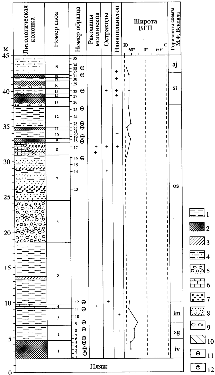
Рис. 3. Литологическая колонка, биостратиграфическая и палеомагнитная характеристики разреза Любимовка. 1–3 – глина и алевро-глина: 1 – светлой окраски, 2 – красно-коричневой окраски, 3 – коричнево-бурой окраски; 4 – алевролит и песчанистая глина; 5 – галечник и конгломерат; 6 – известняк; 7 – гравий; 8 – песок; 9 – карбонатные стяжения; 10 – осыпи и оползни. Намагниченность: 11 – обратная; 12 – неустановленная.
