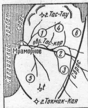
Схема распространения нижне- меловых отложений на север- ном склоне Чатырдага 1 — нижнемеловые отложения на территории Салгирского грабена; 2 — титонские изве- стняки; 3 — тектонические на- рушения (сбросы); 4 — обнаже- ния отложений нижнего мела на северном склоне Чатырдага
