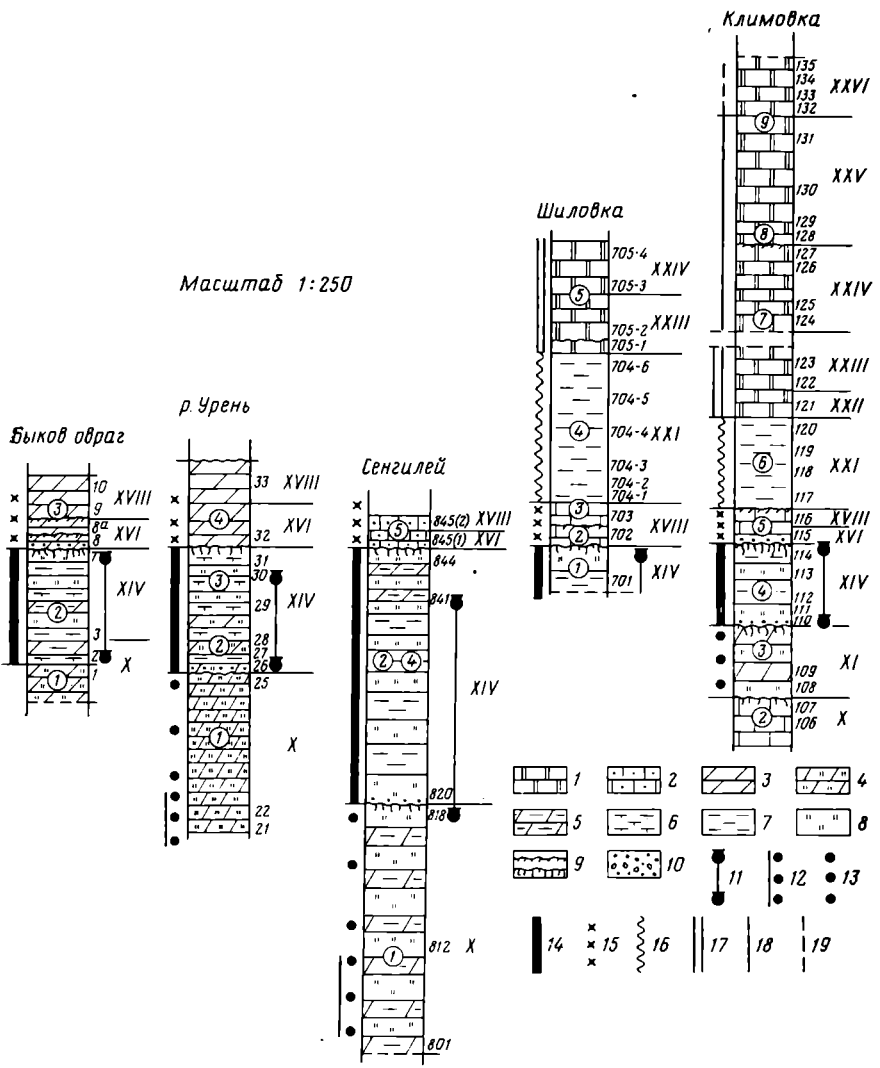
Рис. 2. Фораминиферовые слои и распространение белемнитов. Римские цифры справа от колонок — фораминиферовые слои Мел: 1 — песч. 2 — грубый; мергели: 3 — мелоподобные, 4 — глинистые, 5 — глинистые; глины: 6 — известковые, 7 — неизвестковые; 8 — опоки; 9 — различные образования типа «твердого дна», 10 — гальки. Интервалы распространения: 11 — окситом; 12—19 — белемнитов: 12 — Actinocamax fragilis Arkh. (толстый), Belemnitella cf. propinqua Moberg, 13 — Actinocamax fragilis Arkh. (тонкий), 14 — Actinocamax laevigatus Arkh., Belemnitella ex gr. praecursor Stoll., B. praecursor media Jel., Paractinocamax sp., P. grossouveri cf. alfridi (Janet.), 15 — Paractinocamax sp., P. grossouveri psedotacasi Najdin, Belemnitella mucronata mucronata (Scholt.) Arkh., 16 — Belemnitella langeti Schatsky, 17 — Belemnella lanceolata lanceolata (Schloth.), Bel. lanceolata gracilis (?) (Arkh.), 18 — Belemnella sumensis Jel, 19 — Belemnella sumensis Jel. (очень тонкий ростр), Bel. cf. sumensis Jel.
