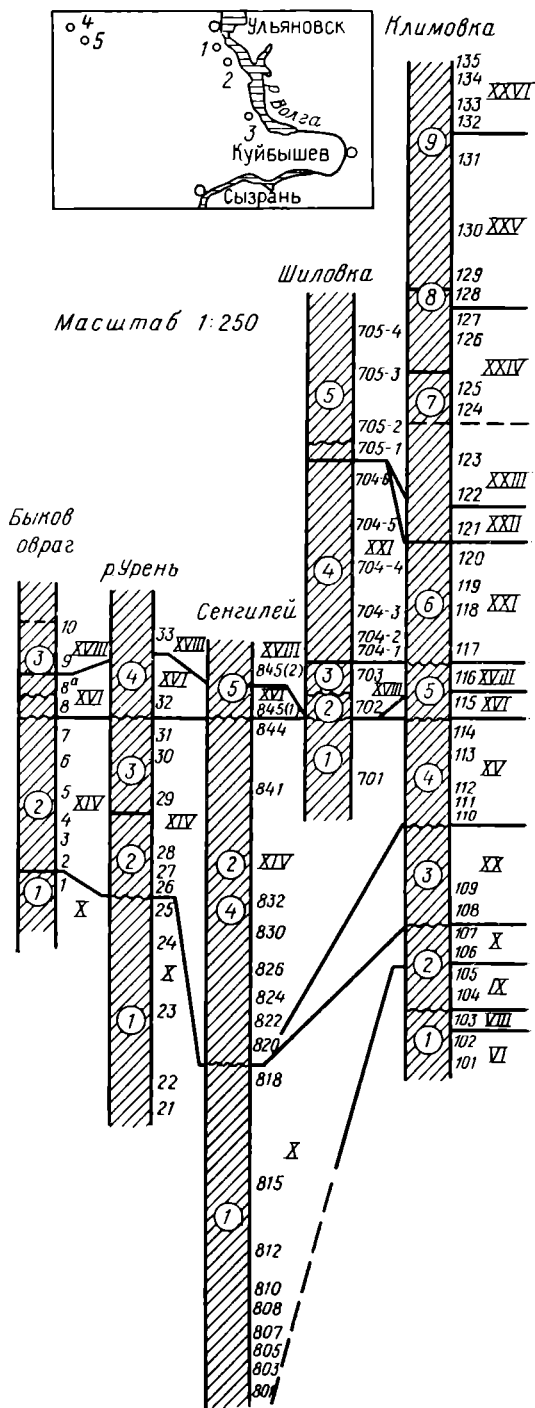
Рис. 1. Расчленение верхнемеловых разрезов Ульяновского Поволжья по фораминиферам На врезке: 1 — Шиловка, 2 — Сенгилей, 3 — Климовка, 4 — Быков овраг, 5 — р. Урень. Арабские цифры на колонках (в кружках) — литологические слои и пачки; арабские цифры справа от колонок — микрофаунистические пробы. Римские цифры — фораминиферовые слои (состав их рассмотрен в тексте)
